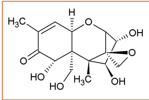
Kuva 4. Nivalenolin rakenne
