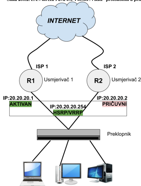
Slika 200.2. LAN mreža s dva ISP-a i HSRP/VRRP protokolom u primjeni
