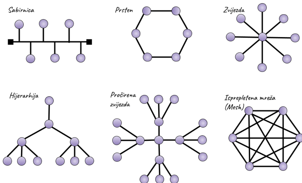
Slika 143. Topologije mreže
