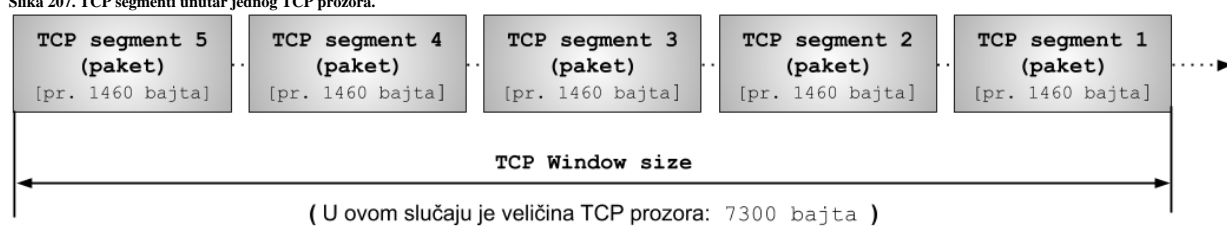
Slika 207. TCP segmenti unutar jednog TCP prozora.
