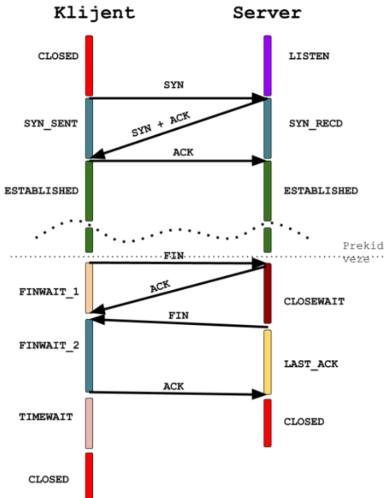
Slika 227. Stanja TCP veze klijenta i poslužitelja.
