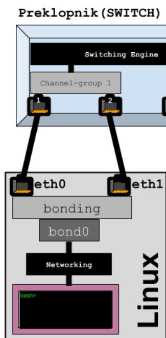
Slika 176. Detaljniji prikaz povezivanja preklopnika s Linuxom.
