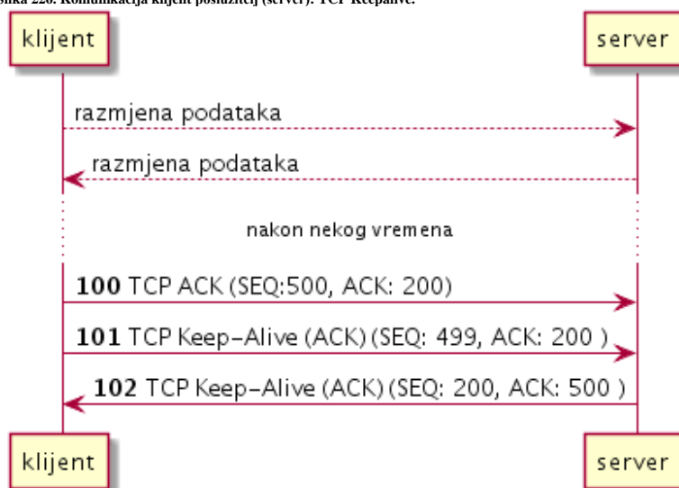
Slika 226. Komunikacija klijent poslužitelj (server): TCP Keepalive .
