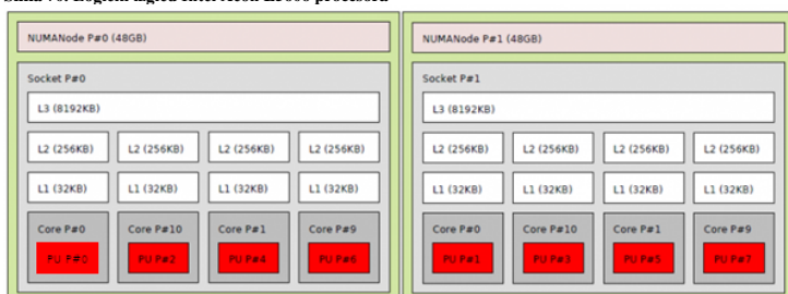
Slika 70. Logički izgled Intel Xeon E5606 procesora
