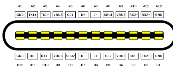
Slika 45.3. USB tip C.
