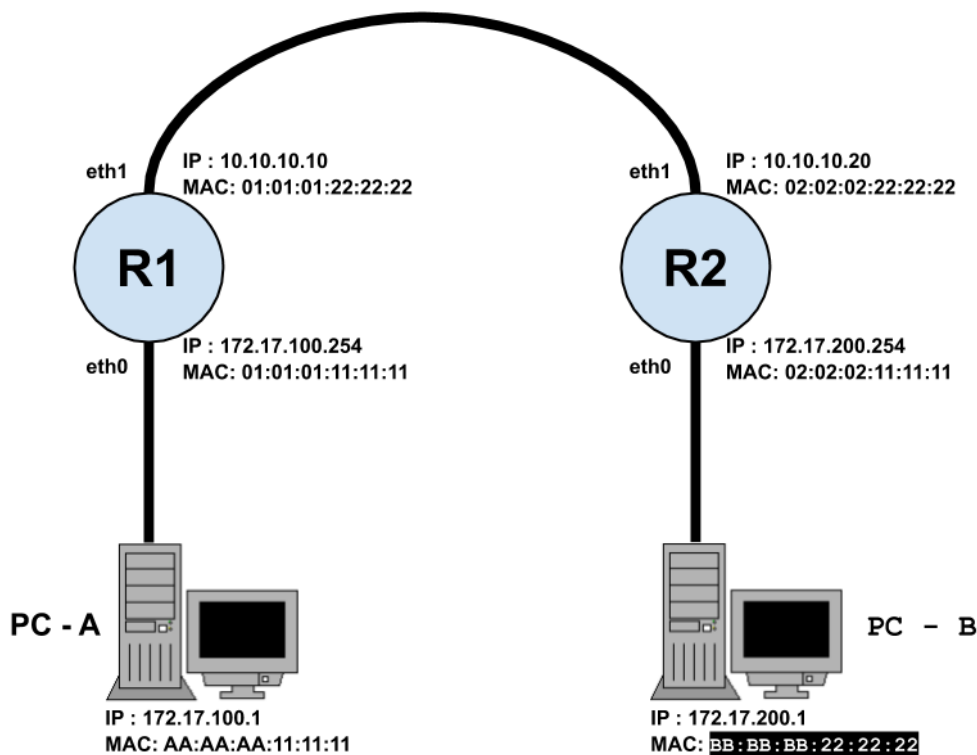
Slika 197. Topologija mreže.
