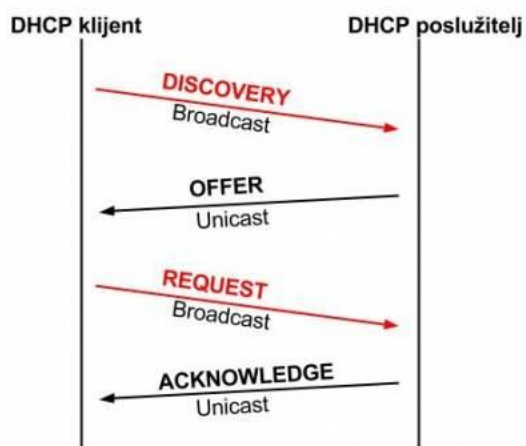
Slika 239. DHCP komunikacija.
