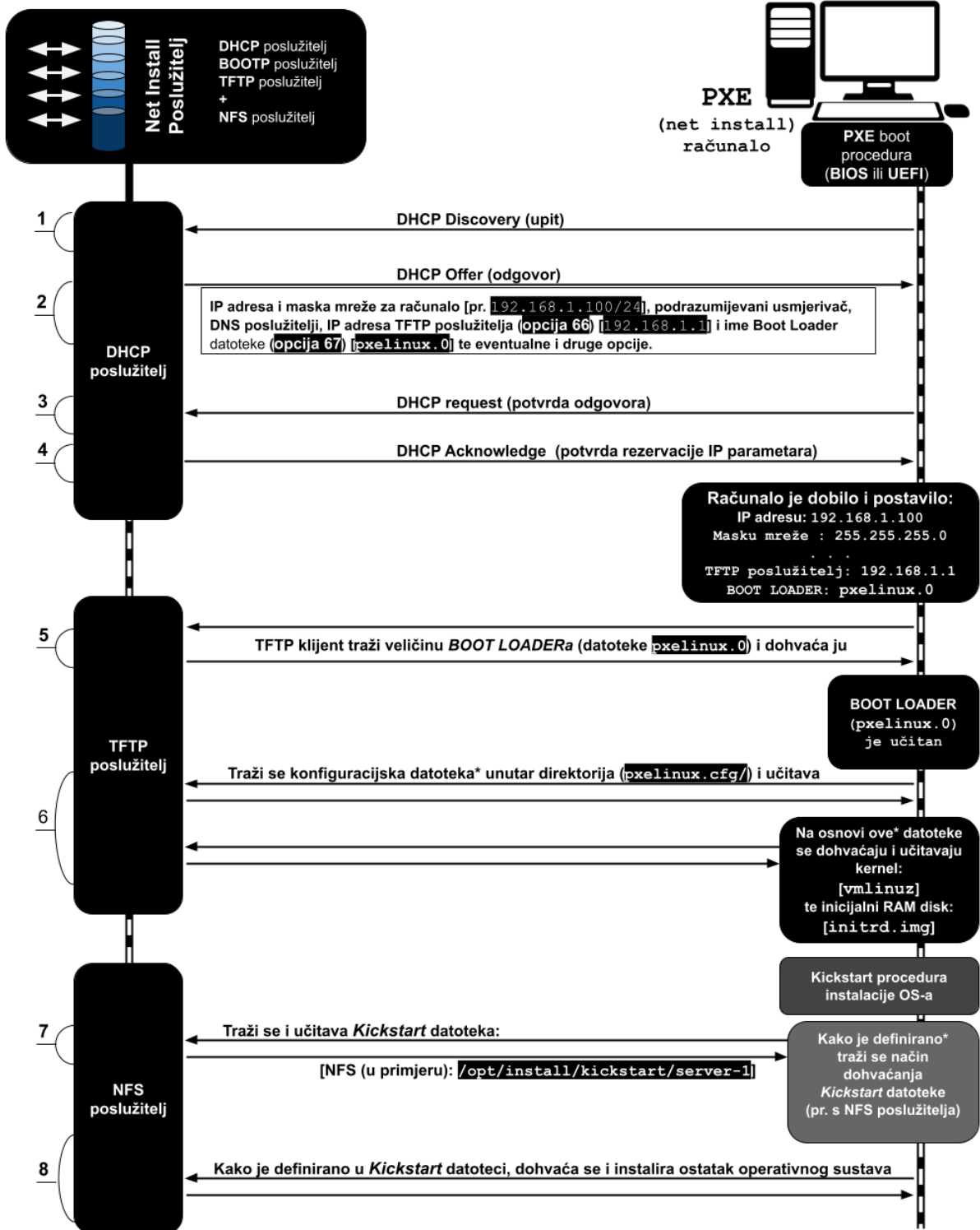
Slika 241.2 PXE boot odnosno network install procedura s mrežnog instalacijskog poslužitelja.
