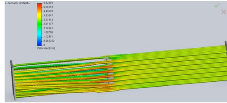
Figura 30: simulación túnel de viento, Rotor Savonius con un ángulo de 45° Fuente: Propia
