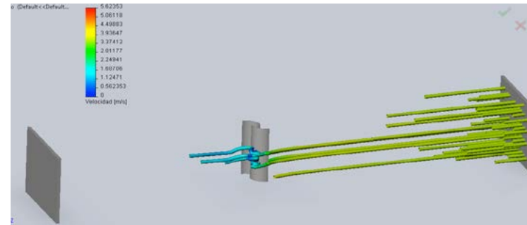
Figura: 31 turbulencias a la salida del viento Fuente: Propia
