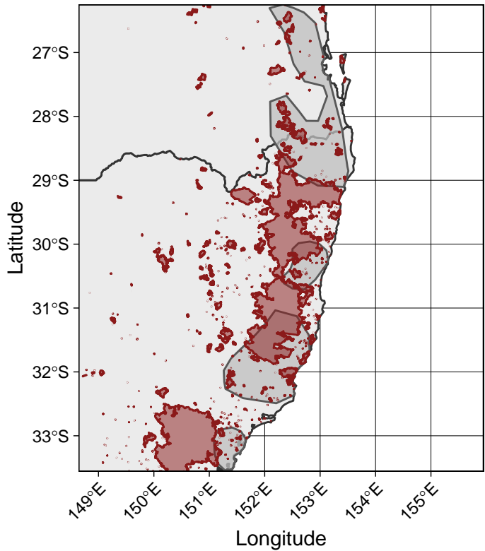
A) Hypsilurus spinipes
