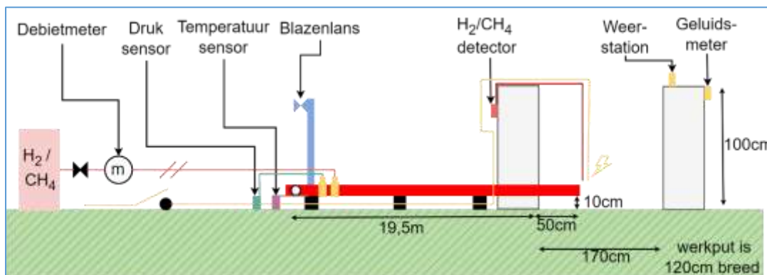
Figuur 3 Meetopstelling directe ontsteking met een buislengte van 20 meter
