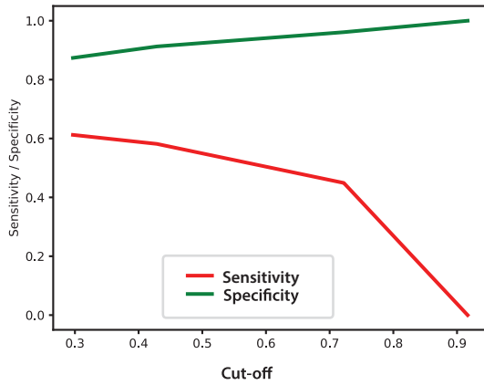
DT
