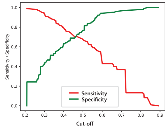
SVM
