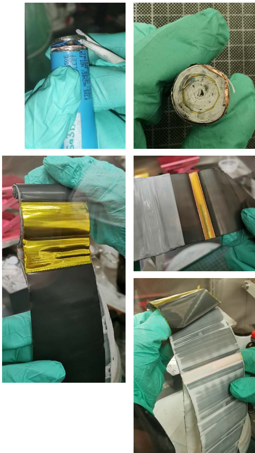
Figure 16. Samsung INR21700-50E
