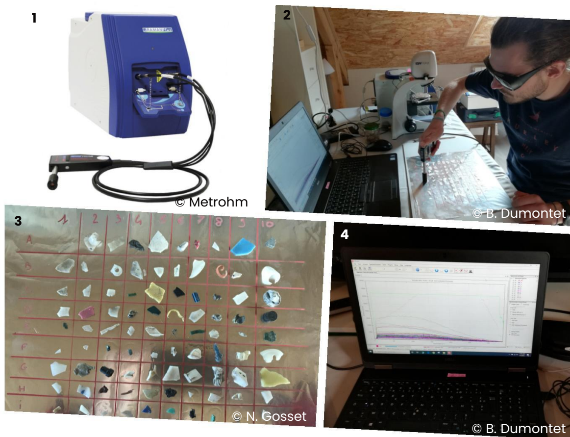
Figure 5 - Analyse Raman des potentiels plastiques issus du m_2 (1 - iRaman plus 785S ; 2 - utilisation de la sonde du raman pour identifier la composition chimique des morceaux ; 3 - mise en place des morceaux avant l'analyse Raman ; 4 - accumulation des spectres sur l'ordinateur)
