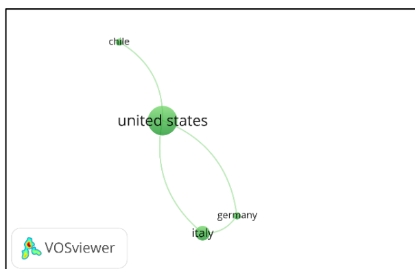
Gráfico 10 – Rede de Países - Cluster 2
