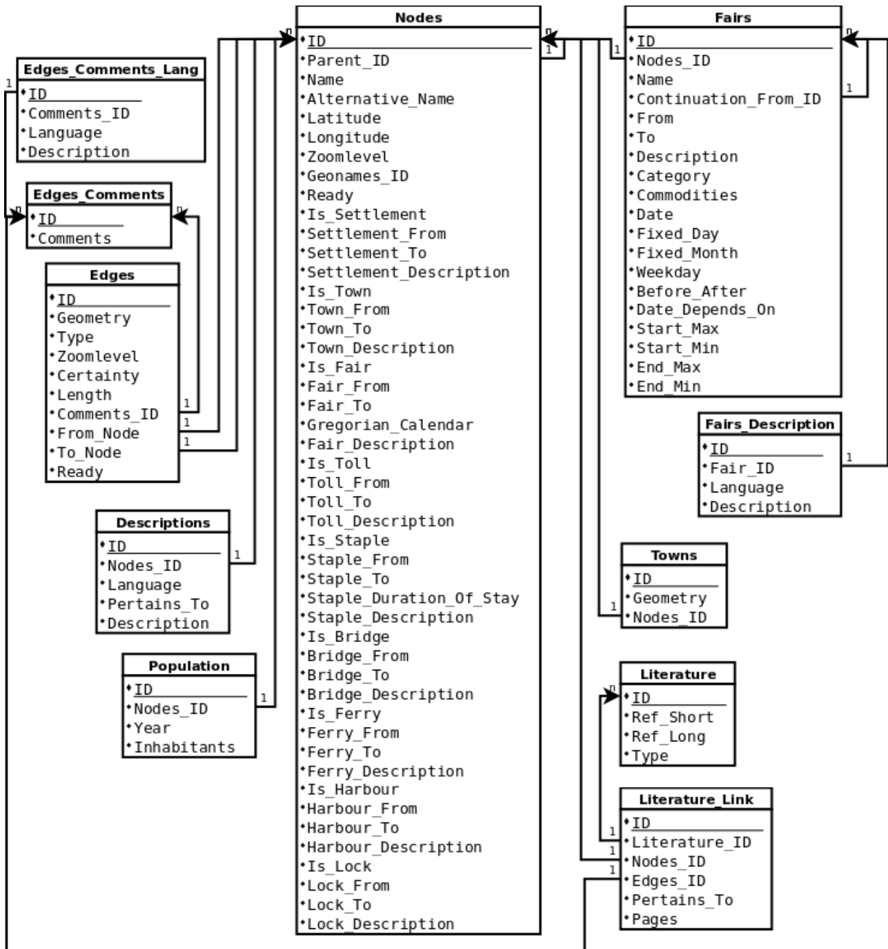
The Viabundus database schema.
