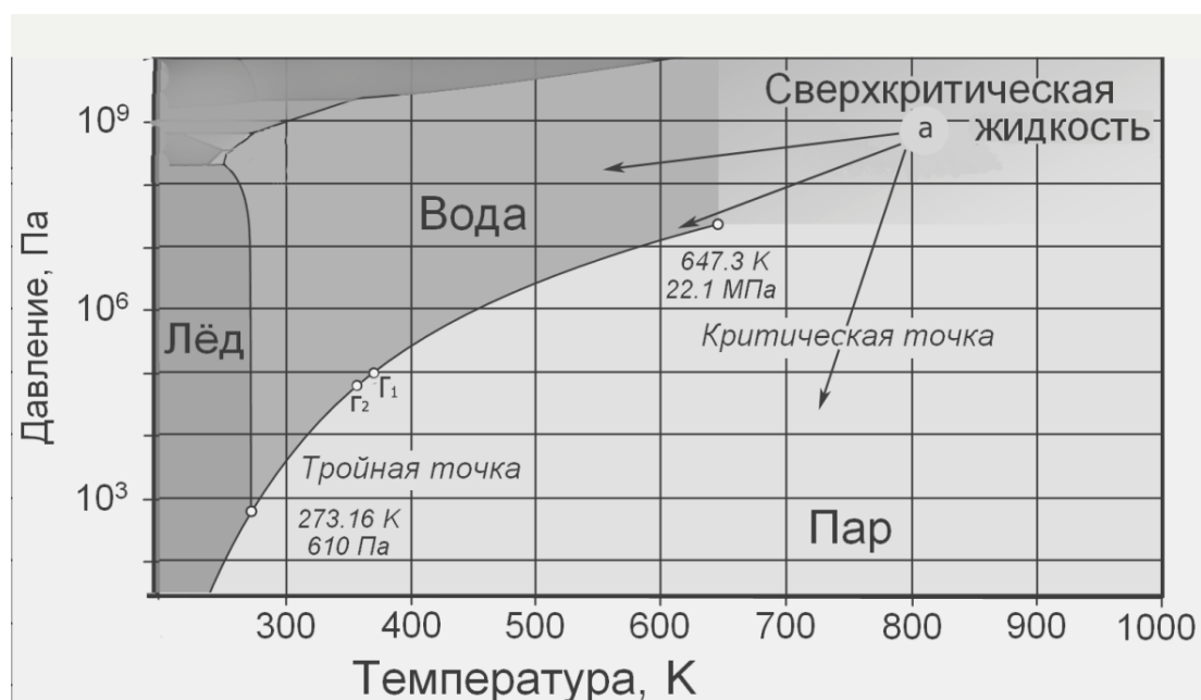
Рис.1. Фрагмент фазовой диаграммы состояния воды по IAPWS. Объяснения – в тексте.
