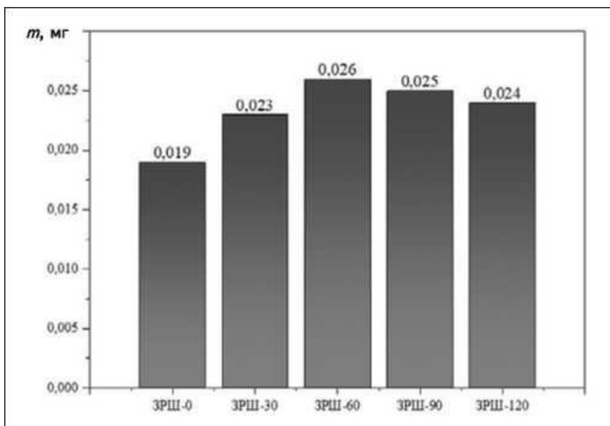
Рис. 1. Масса растворенного оксида кремния, мг, в образцах золы рисовой шелухи с различной продолжительностью механоактивации
