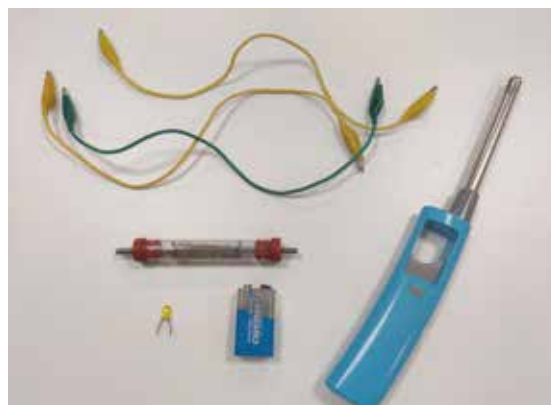
Figura 4. Elementos para el experimento de Branly. (Imagen propia).
