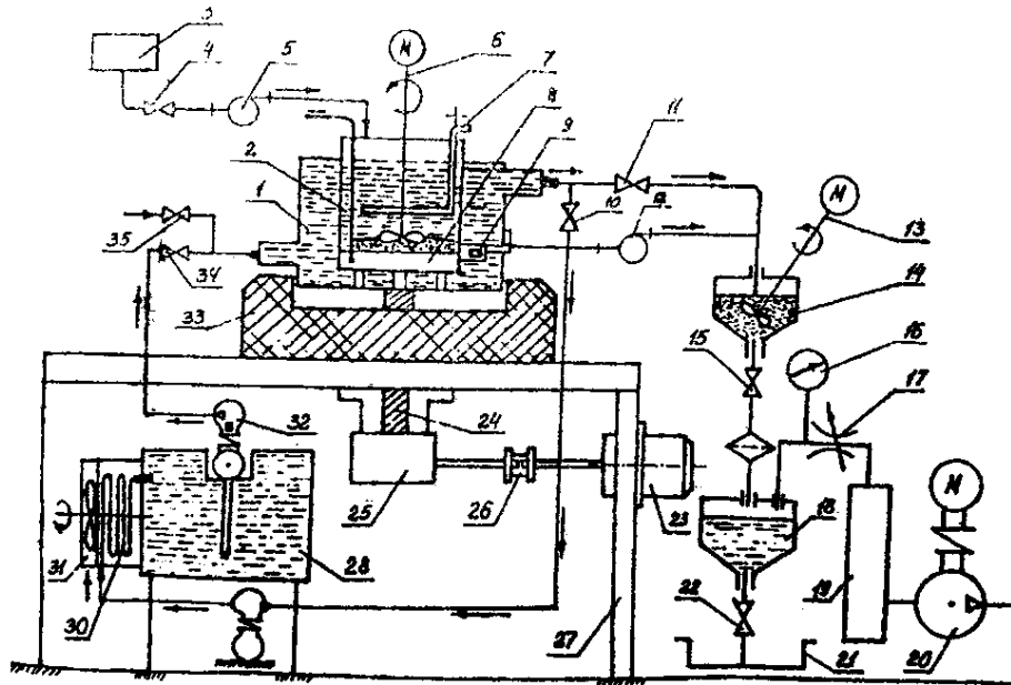
Рис. 3. Экспериментальная установка для проведения исследований.
