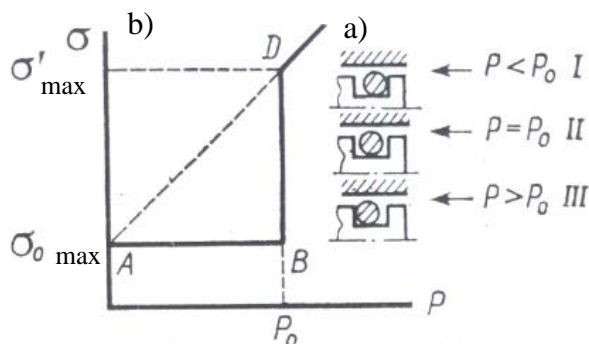
Şəkil 2. Dairəvi enkəsikli həlqənin yuvaya P təzyiği verildiyi vəziyyət (a) və təmas gərginliyinin təzyiqdən asılılığı (b) sxemi.
