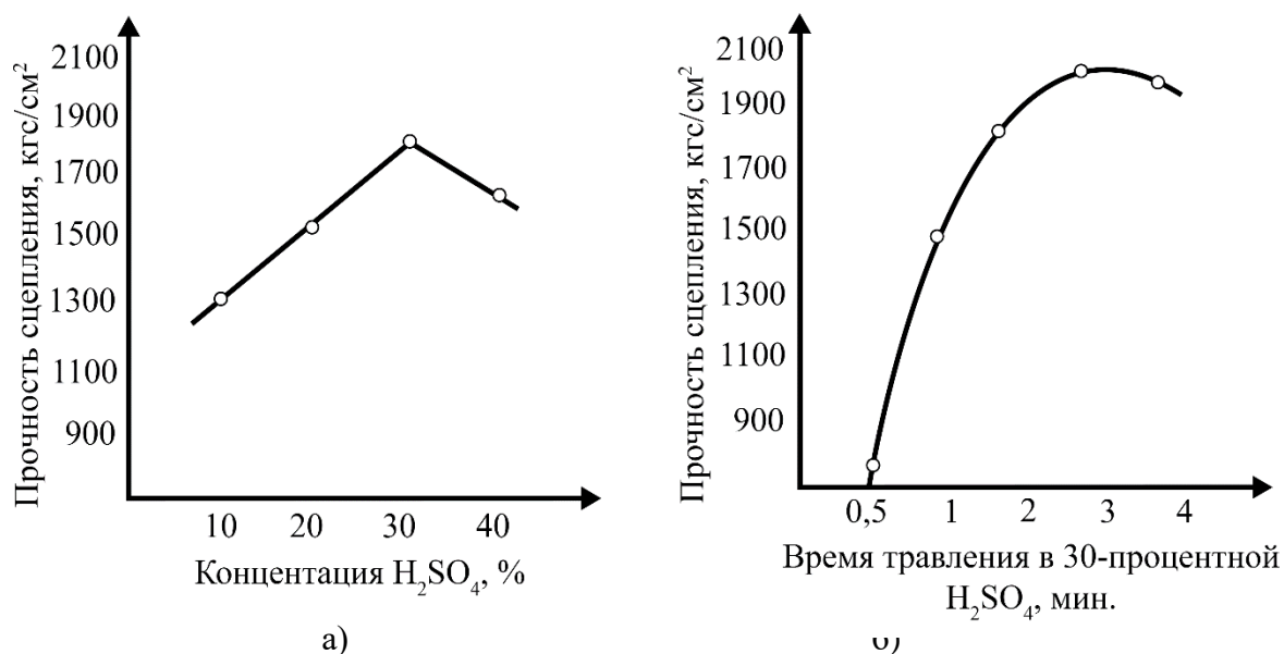
Рис. 7. Зависимость прочности сцепления осадков железа с основным металлом от концентрации H 2 SO 4 при D_a=20\text{а/дм}^2 и T=2\text{мин.} (а) и продолжительности (б) травления.
