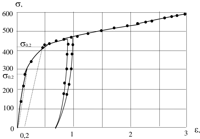
Şəkil 3. Polimer əsaslı kompozisiya tərkibli dairəvi en kəsiyə malik kipgəcin gərginlik-deformasiya diaqramı: – nəzəri; • təcrübi nəticələr
