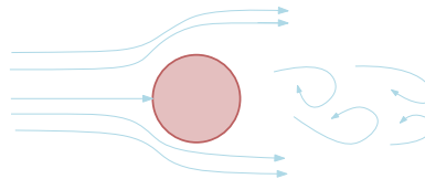
Fig. 9.4 – Oscillating Von Karman Vortex Street.
