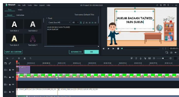
Gambar 3. Pembuatan Tulisan
