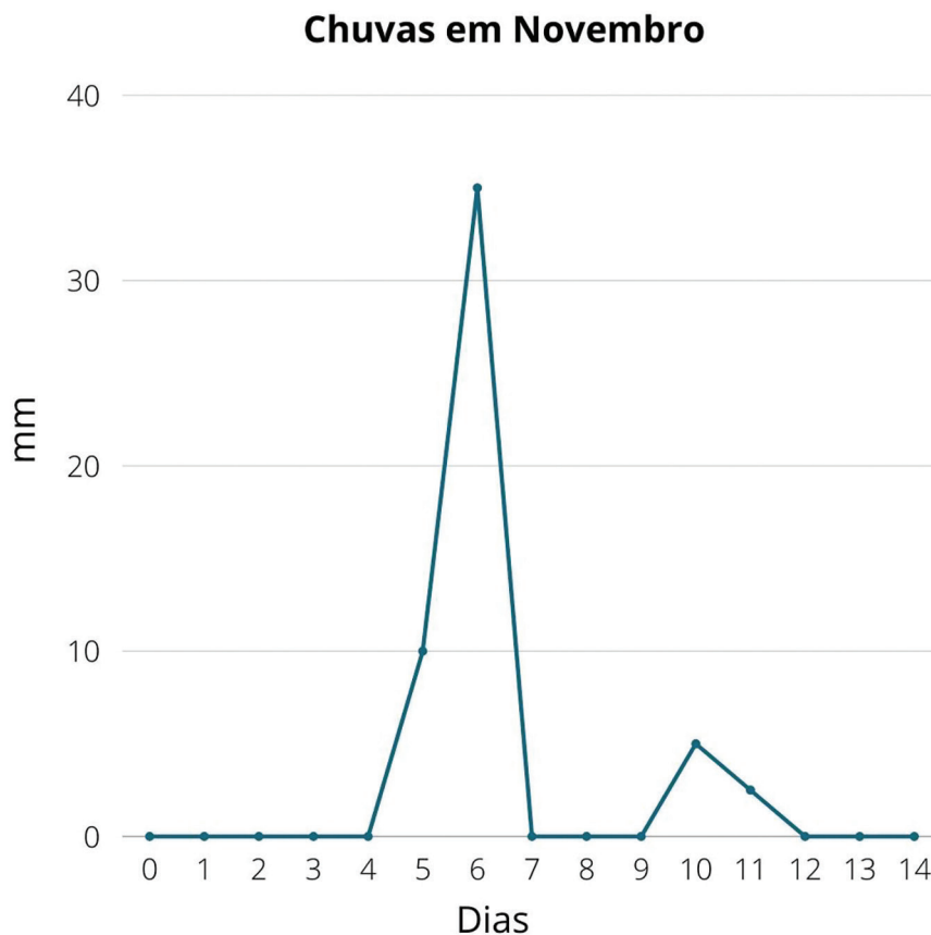
Figura 45 - Gráfico das leituras diárias do pluviômetro artesanal.
