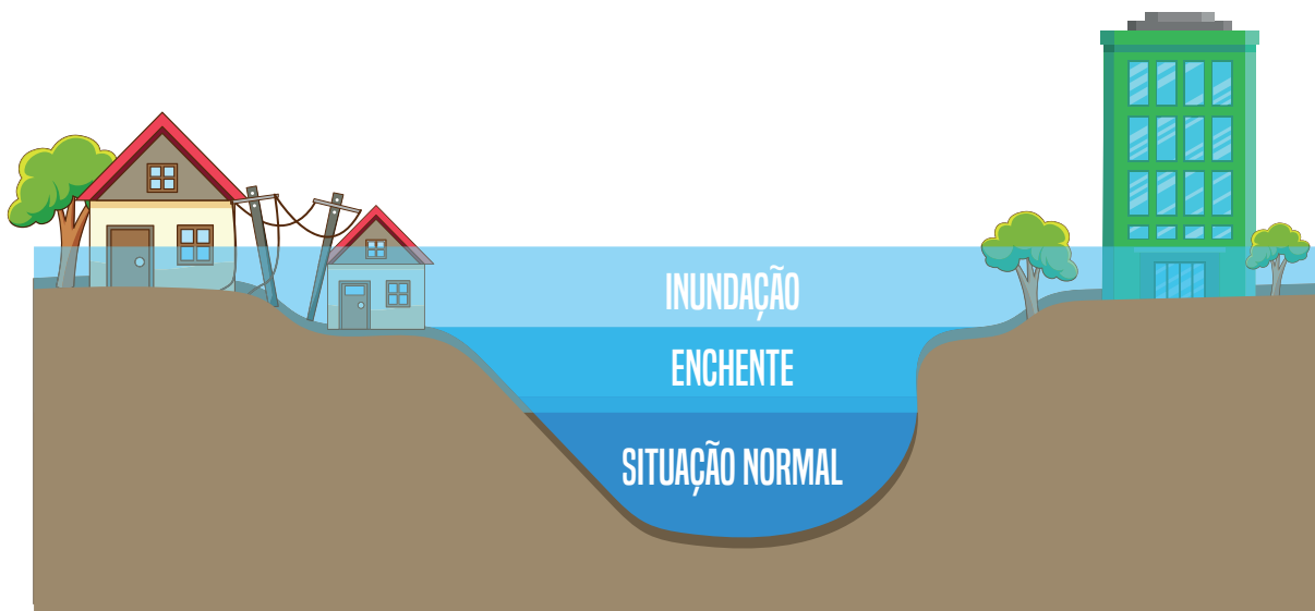
Figura 25 - Relação entre enchentes e inundações.
