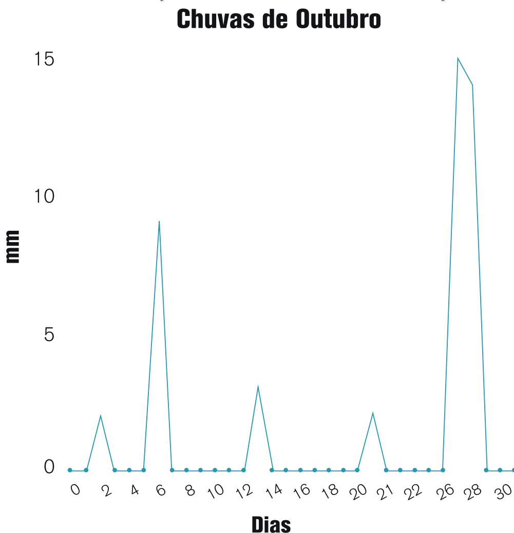
Figura 29 - Quantidade de chuva precipitada no mês de outubro de 2019 em São Paulo, coletada por estudantes da Escola Estadual Vicente Leporace.
