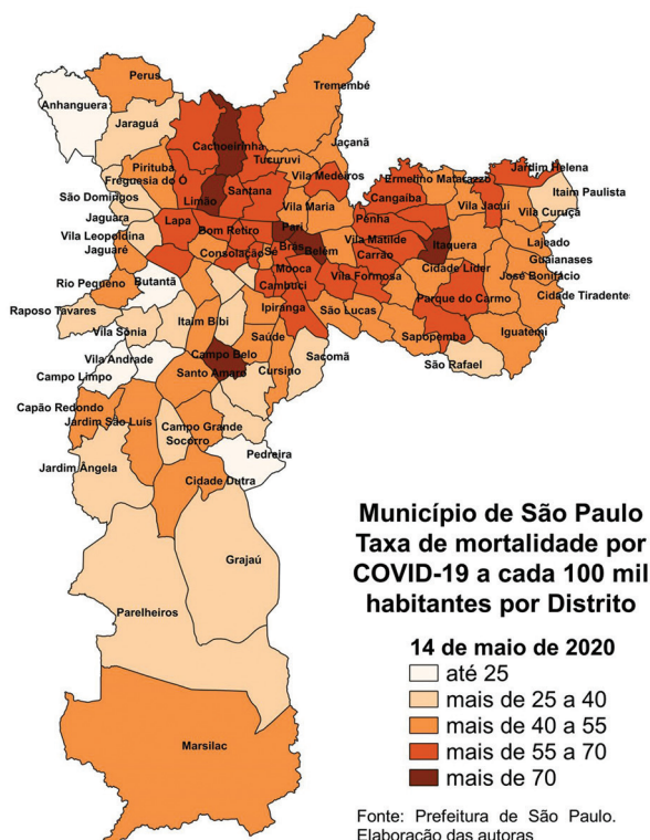
Figura 22 - Mapa da taxa de mortalidade por Covid-19 nos distritos da cidade de São Paulo.
