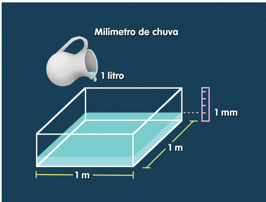
Figura 44 - Representação de lâmina d'água de 1mm de chuva.
