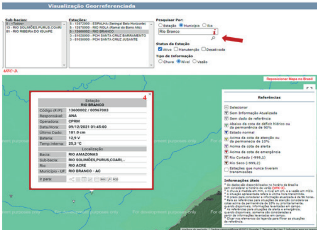
Figura 53 - exemplo de acesso a dados no sistema Hidroweb, tendo como base o município de Rio Branco, AC.
