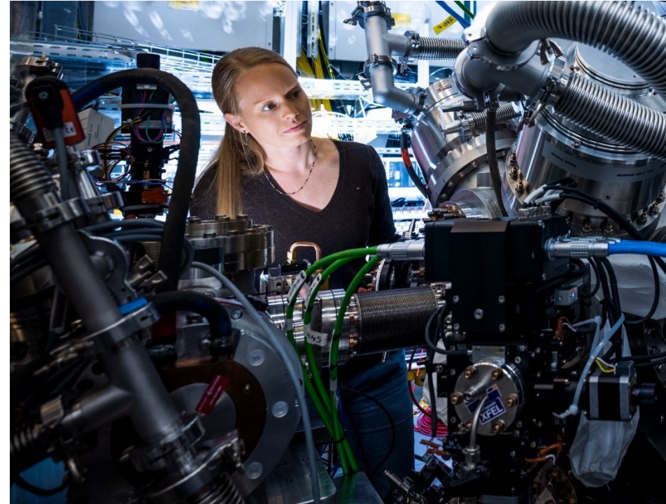
XFEL
