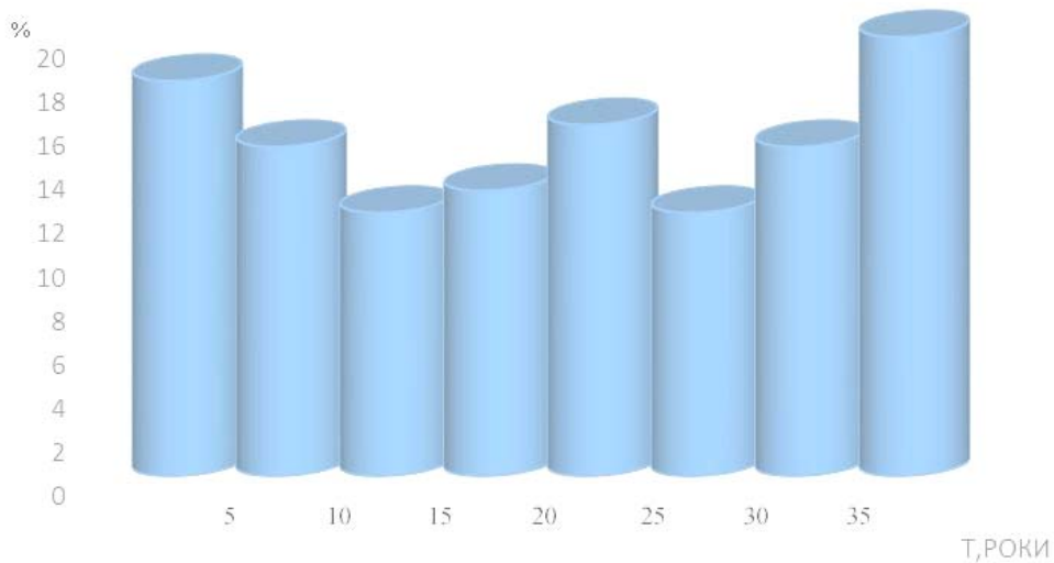
Рис. 5. Розподіл відмов і пошкоджень силових трансформаторів за періодами експлуатації, %
