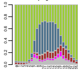
Survey age 25-54
