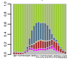
Survey all
