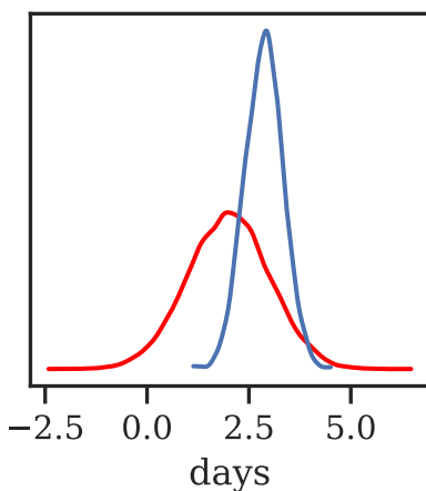
GI sd
