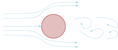
Fig. 9.4 – Oscillating Von Karman Vortex Street.
