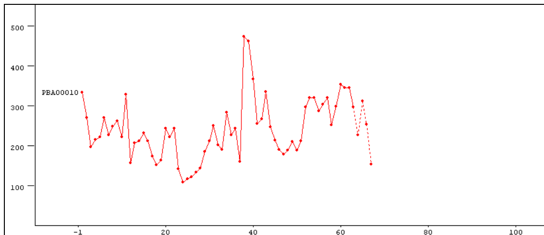
Afbeelding 3. Ongedateerde meetreeks PBA00010 (de gestippelde lijn geeft de spintringen weer); y-as: jaarringbreedte in \text{mm} \cdot 10^{-2} ; x-as: nummer van jaarringen.
