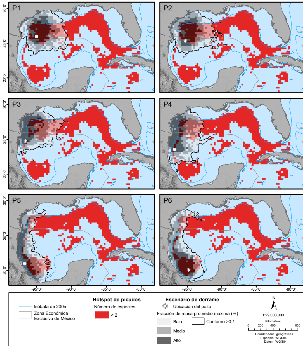
Figura 4. Traslado entre los hotspots de picudos y el área de distribución de la fracción de masa promedio máxima de petróleo pesado de cada escenario de derrame (del P1 al P6). Los hotspots (área roja) son las áreas en donde coinciden \geq 2 especies.
