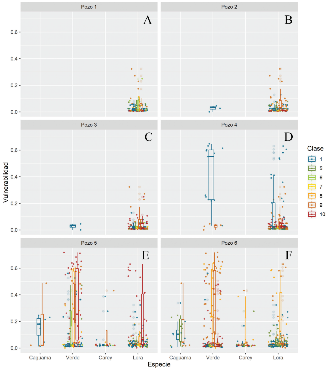
Figura 8. Representación de la variabilidad de la interacción entre los escenarios de derrames de hidrocarburo para los seis pozos (A-) representado como categorías de severidad (integración P_{max} y T_{hit} ) y la vulnerabilidad ecológica acumulada de cada especie de tortuga marina. En la gráfica de cada pozo, los puntos de colores (categorías de severidad del derrame) representan la cantidad de hexágonos que interactuaron con el escenario de derrame, mientras que las cajas con bigotes expresan las estadísticas de la vulnerabilidad para categoría de severidad, y su anchura está asociada a la cobertura geográfica de la interacción (número de puntos/hexágonos), diferenciado por especie de tortuga marina.
