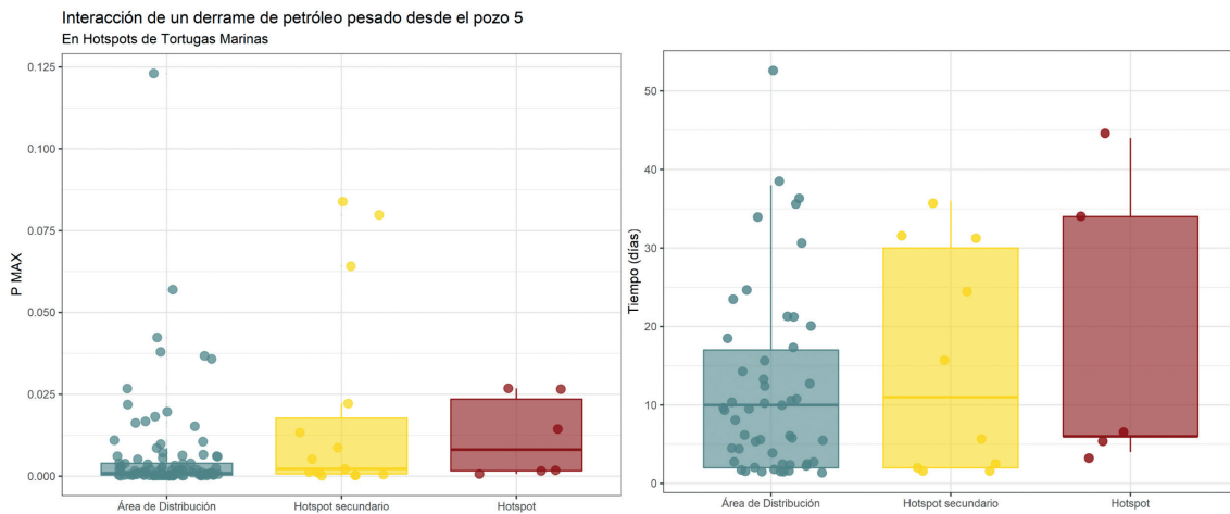
Figura S4. Síntesis gráfica de los valores (puntos) y las estadísticas (cajas y bigotes) de la interacción entre las variables del escenario de derrame, la fracción de masa promedio máxima de hidrocarburo ( P_{max} ) para un área dada (A) y el tiempo de arribo ( T_{hit} ) al área de interés (B), con la ubicación de los Hotspots de cuatro especies de tortugas marinas residentes del golfo de México y Caribe mexicano.
