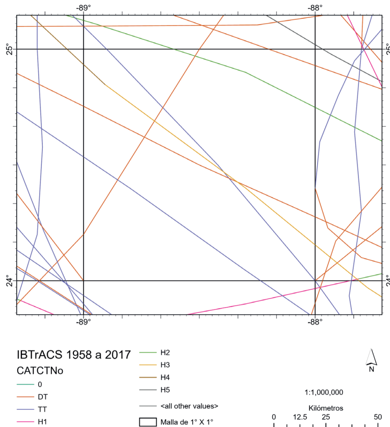
Figura 9. Malla usada para contar el número de ciclones tropicales por categoría para el cálculo de las excedencias.
