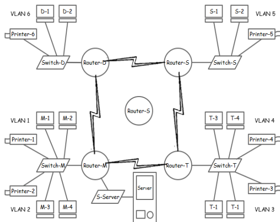
Gambar.1 Desain VLAN
