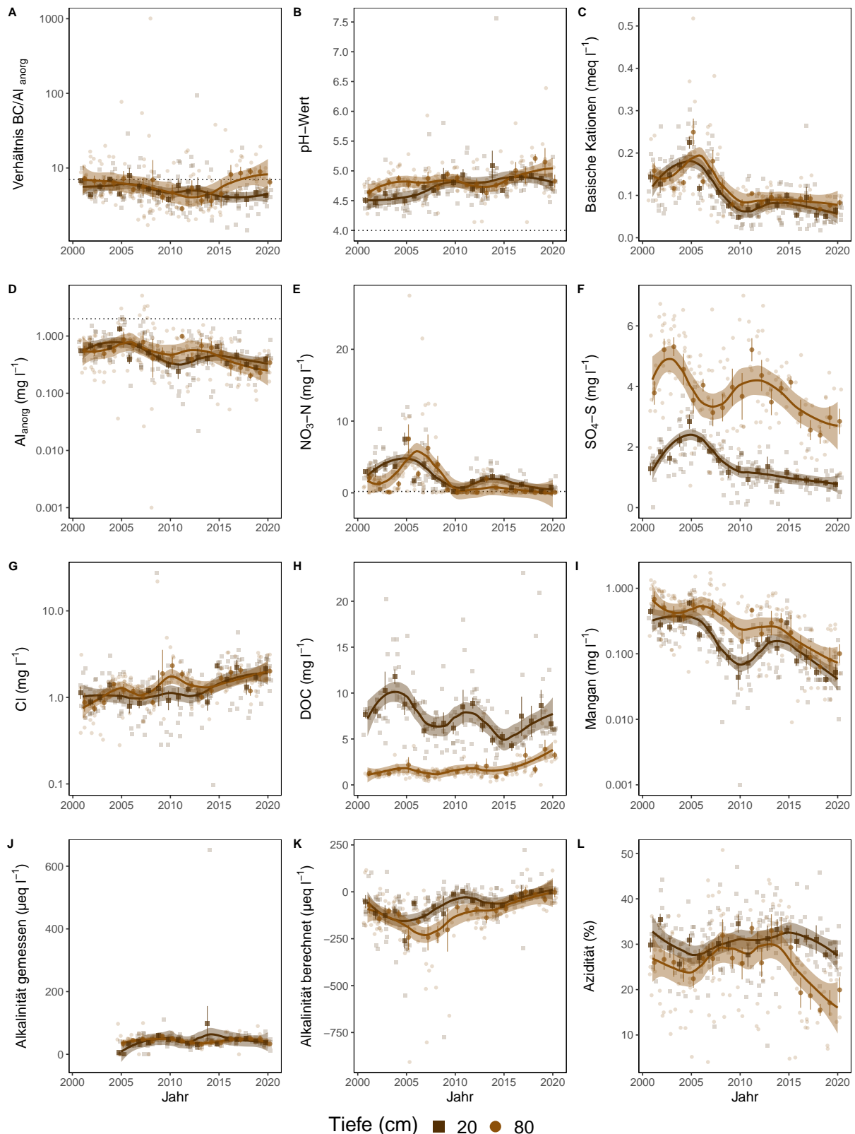
Abb. 86. Entwicklungen in der Bodenlösung der Beobachtungsfläche Habsburg (AG) Lotharfläche Kontrolle Buchen. A) BC/Al-Verhältnis mit Grenzwert als Punktlinie ( (BC/Al)_{crit} \leq 7 ), B) pH-Wert mit Grenzwert \leq 4 , C) basische Kationen (BC), D) Aluminium anorganisch mit kritischer Konzentration \geq 2 \text{ mg l}^{-1} , E) Nitratstickstoff mit Grenzwert für Vegetationsveränderungen \geq 0.2 \text{ mg l}^{-1} , F) Sulfatschwefel, G) Chloridkonzentration, H) gelöster organischer Kohlenstoff (DOC), I) Mangankonzentration, J) gemessene Alkalinität, K) berechnete Alkalinität (ANC) L) Azidität. Dargestellt sind die monatlichen Messungen und Jahresmittelwerte mit Standardfehler als Linie. Der zeitliche Trend ist mit einer local polynomial regression fitting (Loess, \alpha=0.5 ) Funktion dargestellt.
