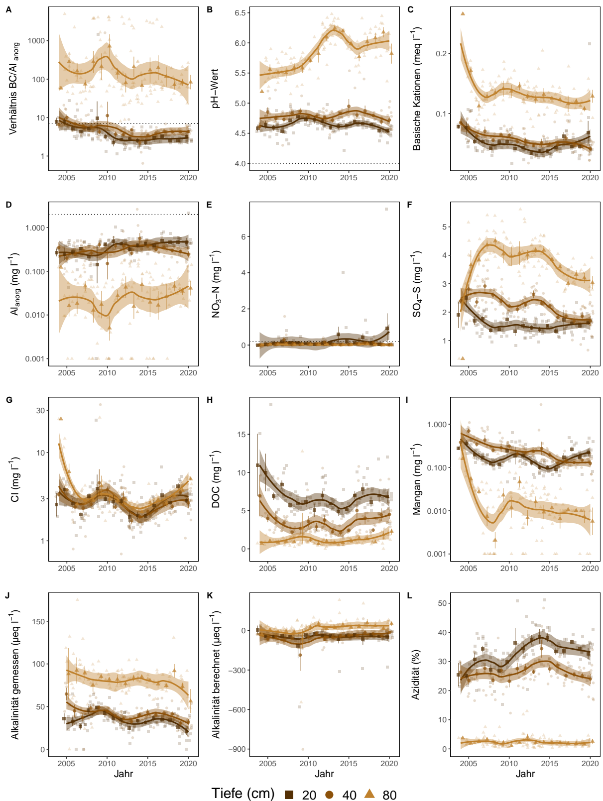
Abb. 106. Entwicklungen in der Bodenlösung der Beobachtungsfläche Olsberg (AG) Buchen. A) BC/Al-Verhältnis mit Grenzwert als Punktlinie ( (\text{BC}/\text{Al})_{\text{crit}} \leq 7 ), B) pH-Wert mit Grenzwert \leq 4 , C) basische Kationen (BC), D) Aluminium anorganisch mit kritischer Konzentration \geq 2 \text{ mg l}^{-1} , E) Nitratstickstoff mit Grenzwert für Vegetationsveränderungen \geq 0.2 \text{ mg l}^{-1} , F) Sulfatschwefel, G) Chloridkonzentration, H) gelöster organischer Kohlenstoff (DOC), I) Mangankonzentration, J) gemessene Alkalinität, K) berechnete Alkalinität (ANC) L) Azidität. Dargestellt sind die monatlichen Messungen und Jahresmittelwerte mit Standardfehler als Linie. Der zeitliche Trend ist mit einer local polynomial regression fitting (Loess, \alpha=0.5 ) Funktion dargestellt.
