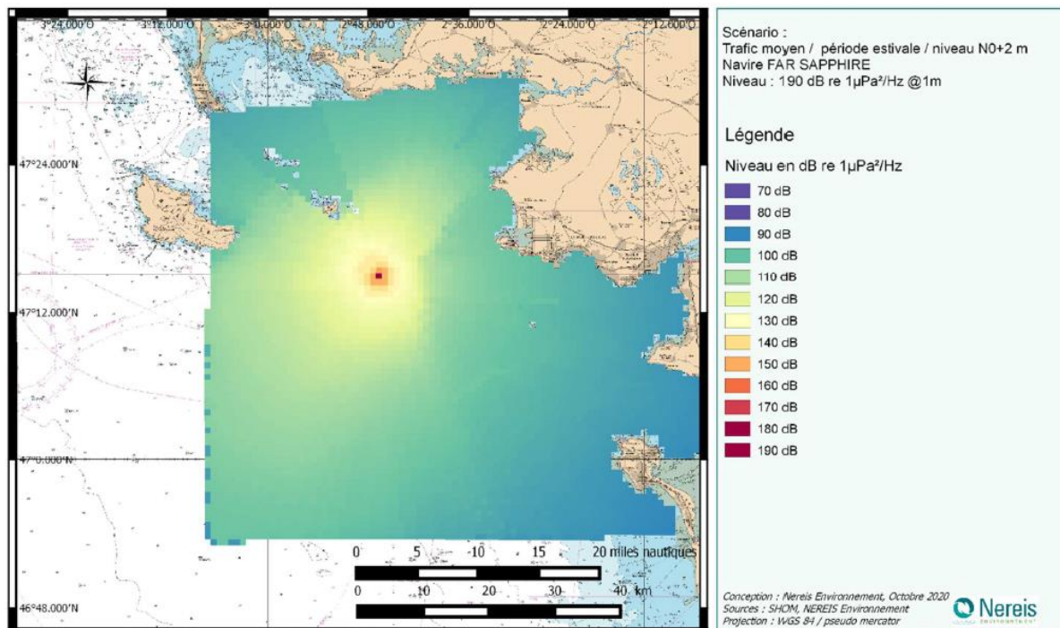
FIGURE 17 : CARTE DU NIVEAU DE BRUIT AMBIANT ASSOCIE A LA PHASE DE MISE EN TENSION DES LIGNES D'ANCRAGE (NIVEAU DE BRUIT LARGE BANDE (7 HZ – 100 KHZ) MAXIMUM A 190 DB REF 1µPA²/HZ@1M - NEREIS ENVIRONNEMENT, 2017).
