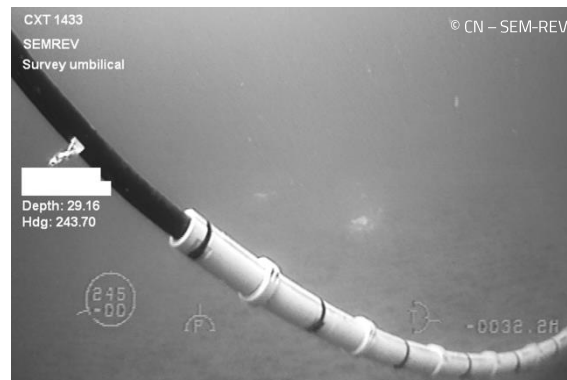
FIGURE 9 : PHOTOGRAPHIE DU CÂBLE OMBILICAL DE L'ÉOLIENNE FLOATGEN - SECTION DU POINT DE TOUCHE AVEC LE FOND MARIN.
