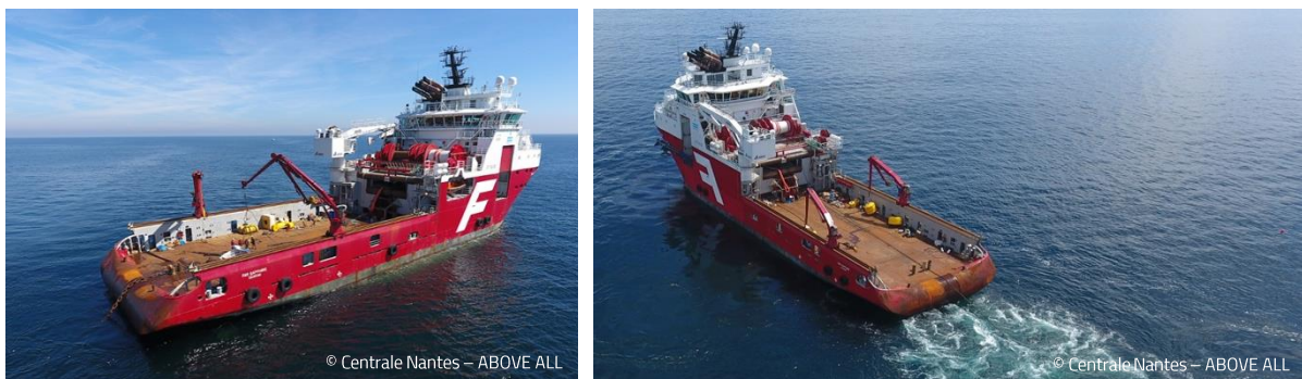
FIGURE 8 : INSTALLATION DES LIGNES D’ANCRAGES DE L’EOLIENNE FLOATGEN.
