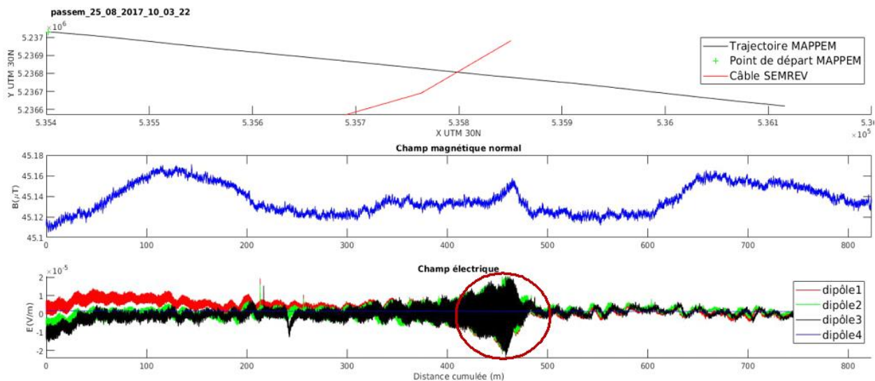
FIGURE 22 : LE CHAMP MAGNÉTIQUE TOTAL ( \mu\text{T} ) ET LES CHAMPS ÉLECTRIQUES ( \text{V}/\text{M} ) MESURÉS (MAPPEM GEOPHYSICS, 2019).
