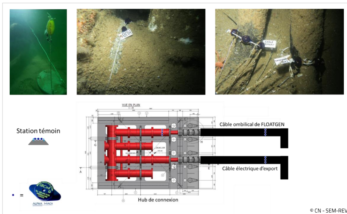
FIGURE 26 : STRATEGIE D'ECHANTILLONNAGE POUR LE SUIVI DE LA TEMPERATURE SUR LES INFRASTRUCTURES ELECTRIQUES DE SEM-REV.
