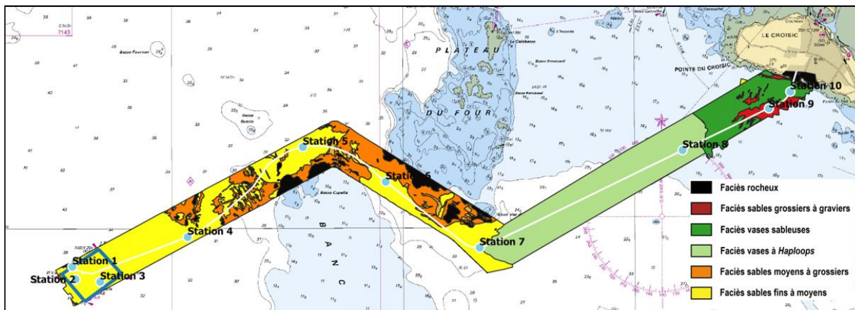
FIGURE 32 : LOCALISATION DES STATIONS DE SUIVI DES COMMUNAUTÉS BENTHIQUES SUR LE SITE D'ESSAIS SEM-REV ET LE LONG DU CABLE DE RACCORDEMENT ELECTRIQUE AVEC LES FACIES SEDIMENTAIRES ASSOCIES (ASTERIE, 2008 & 2010 MIS A JOUR CN - SEM-REV, 2018).
