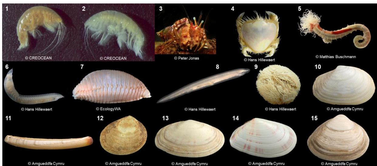
FIGURE 34 : ESPECES D'INTERET ECOLOGIQUE IDENTIFIEES SUR LE SITE D'ESSAIS.
