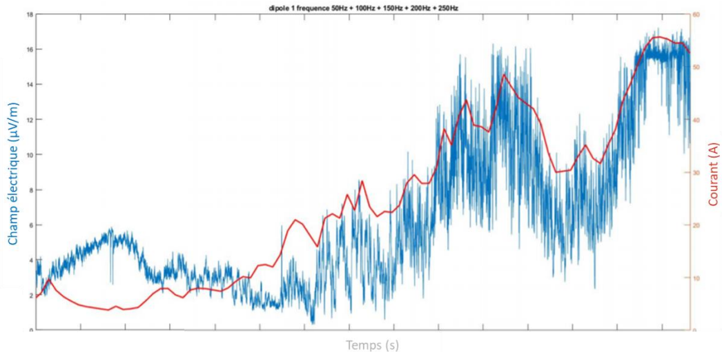
FIGURE 25 : CHAMP ELECTRIQUE ENREGISTRE SUR LE SITE SEM-REV AUX HARMONIQUES PRINCIPALES DU RESEAUX ELECTRIQUE DURANT 17H (EN BLEU) ET INTENSITE DU COURANT DANS LE CABLE (EN ROUGE) (MAPPEM GEOPHYSICS DANS TAORMINA ET AL. , 2020B).
