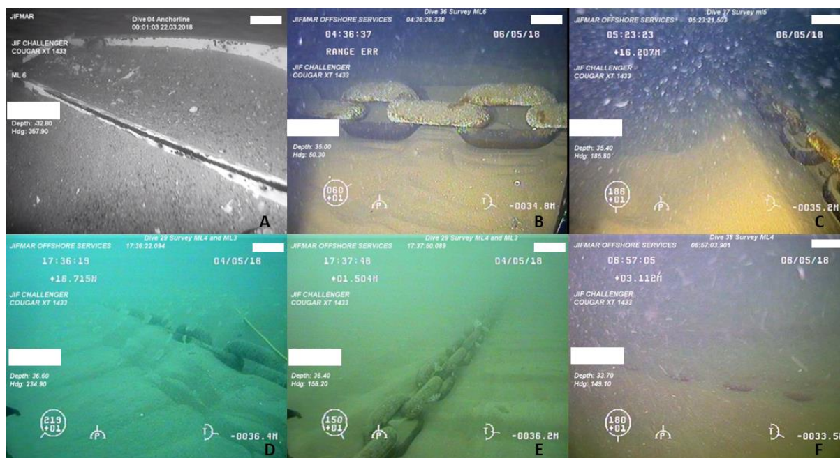
FIGURE 37 : CAPTURES D'ECRANS DES VIDEOS D'INSPECTIONS DES LIGNES D'ANCRAGE DE FLOATGEN. Ces images ont été prises à l'aide d'un R.O.V. en mars et mai 2018 ; A : Ancre de la ligne d'ancre n°6 inspectée en mars 2018 ; B : Chaîne de la ligne d'ancre n°6 inspectée en mai 2018. C : Chaîne de la ligne d'ancre n°5 inspectée en mai 2018 ; D à F : Chaîne de la ligne d'ancre n°4 inspectée en mai 2018 (© BW Ideol & CN – SEM-REV).
