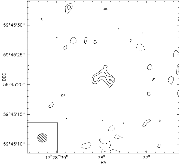
FIG. 5.1 – Contour de densité de flux à 1.4 GHz de la source SDSS J172837.98+594521.5. Les contours sont des multiples de 15 \mu\text{Jy} (-2, 2, 3, 4, 5). Le lobe synthétisé ( 1''.7 \times 1''.5 avec un angle de -30^\circ ) est indiqué dans le coin inférieur gauche de la carte.
