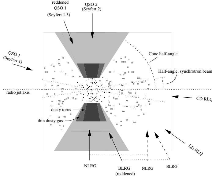
FIG. 2.1 – Modèle d'unification proposé par Wills (1999). Les différentes classes d'AGN dépendent de l'inclinaison par rapport à la ligne de visée du tore de poussière entourant le même moteur central .
