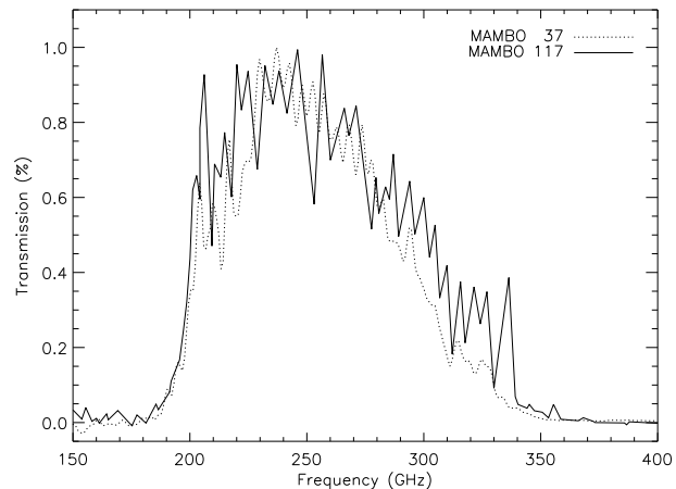
FIG. 3.1 – Droite : Photo de la matrice de bolomètres à 117 canaux MAMBO II. Gauche : réponse spectrale de la matrice de bolomètres MAMBO I & II. Dans les deux cas, la fréquence effective d'observation est 250 GHz.
