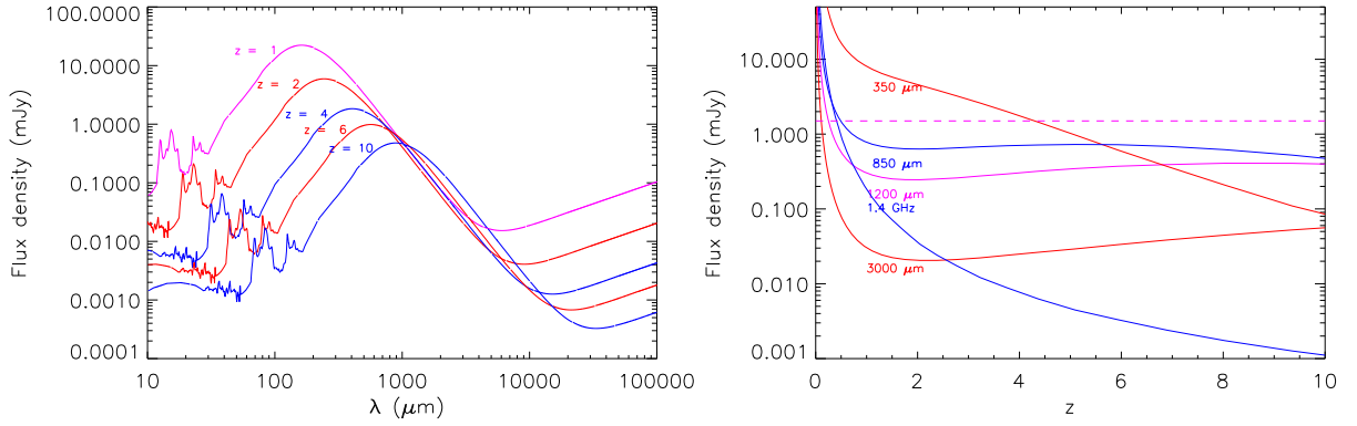
FIG. A.2 – Gauche : Spectre typique d’une galaxie à flambée d’étoile avec L_{\text{FIR}} \approx 10^{12}M_{\odot} observée à différents décalages spectraux. Aucune évolution temporelle n’est appliquée. On peut remarquer pour une longueur d’onde donnée, différents décalages spectraux sondent la distribution spectrale d’énergie à différentes longueurs d’ondes. Droite : Illustration de l’effet de k-correction inverse pour différentes longueurs d’ondes. Le flux d’une galaxie typique à flambée d’étoile à une certaine longueur d’onde observée est reporté en fonction du décalage spectral
