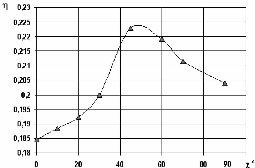
Рис. 4. График зависимости коэффициента тепловой эффективности при задании различных углов входа потока воздуха \chi от 0^\circ (положение закрыто) до 90^\circ (открыто) и относительном расходе Q_a/Q_w=1,1 . Точки – данные численного расчета.
