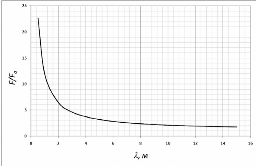
Рис.2. Расчет динамического воздействия на плоскую преграду на пути волны перемещения с дисперсионной зависимостью скорости от длины волны. Скорость течения реки Vn=2,9\text{ м/с} , высота волны 8,4\text{ м} , коэффициент сопротивления 10\text{ м}^2/\text{с} , начальный расход Q=1800\text{ м}^3/\text{с} .
