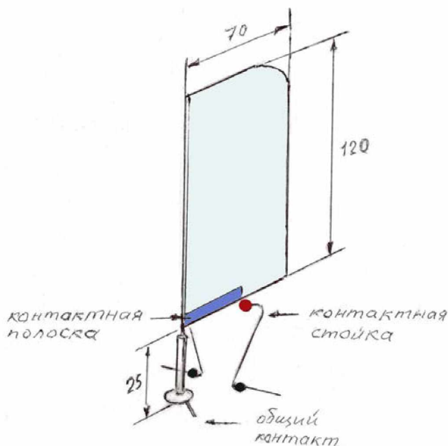
Рис. 8. Схема установленного на катамаране флогера.
