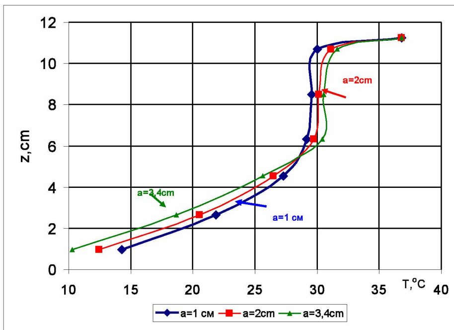
Рис. 6. Вертикальные профили температур внутри сифонного отсека под местом расположения водозаборного шланга при различных высотах открытия целевого затвора.
