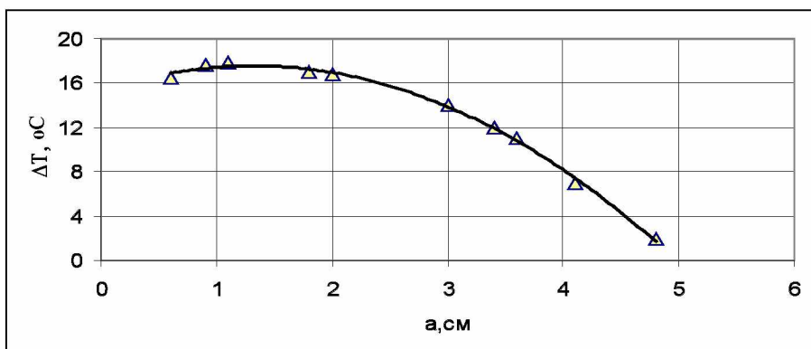
Рис. 7. Зависимость глубины охлаждения оборотной воды от высоты целевого затвора в сифонном отсеке бассейна-охладителя.
