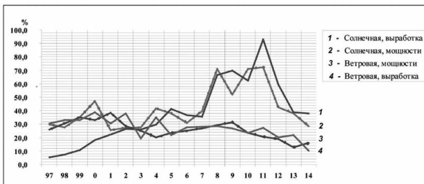
Рис. 1. Динамика годовых темпов роста установленных мощностей и выработки электроэнергии на солнечных и ветряных электростанциях мира в 1997-2014 гг. Источник: BP Statistical Review of World Energy, 2015.
