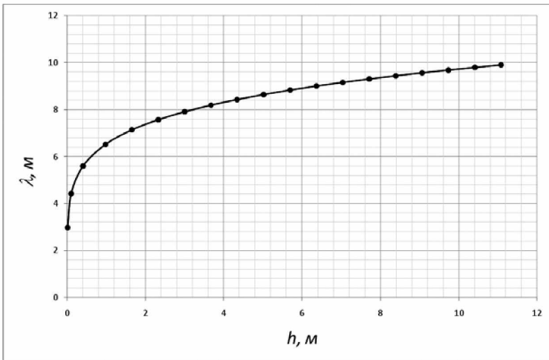
Рис.3. Расчетная зависимость длины волны \lambda_y от высоты волны перемещения h с исходным начальным расходом воды Q=1800\text{ м}^3/\text{с} . Обозначения: круглые маркеры – расчет по уравнениям Сен-Венана неустановившихся движений воды в открытых потоках, сплошная линия – тренд по формуле \lambda = 6.5623h^{0.1715}
