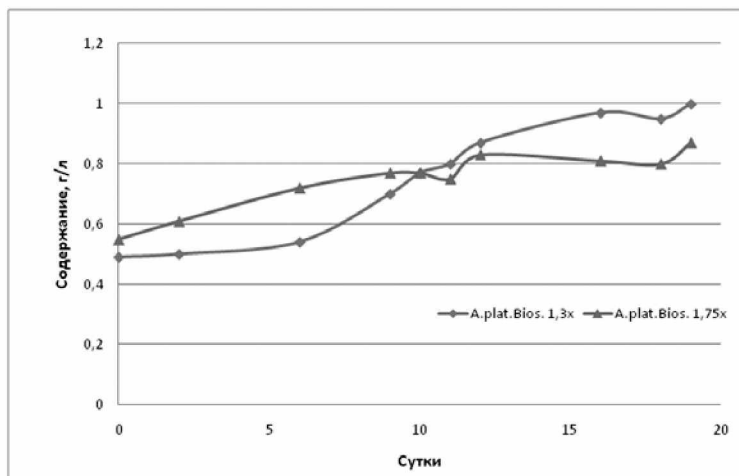
Рис. 3. Продолжение эксперимента: рост клеток A. platensisBios(P) в сточных водах с добавлением дополнительной порции сточных вод после 12 суток роста
