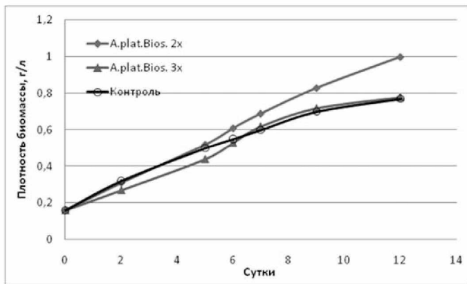
Рис. 2. Динамика плотности биомассы A. platensisBios(P) в сточных водах с 2х и 3х разбавлением
