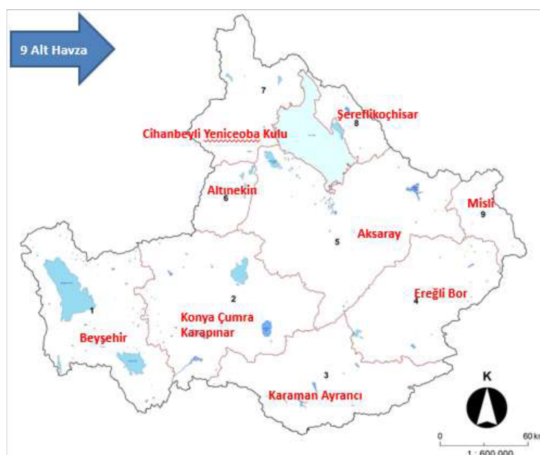
Figure 8. Konya Closed Basin (and sub-basin) borders (T.C. Tarım ve Orman Bakanlığı Su Yönetimi Genel Müdürlüğü, 2018, p. 11)
