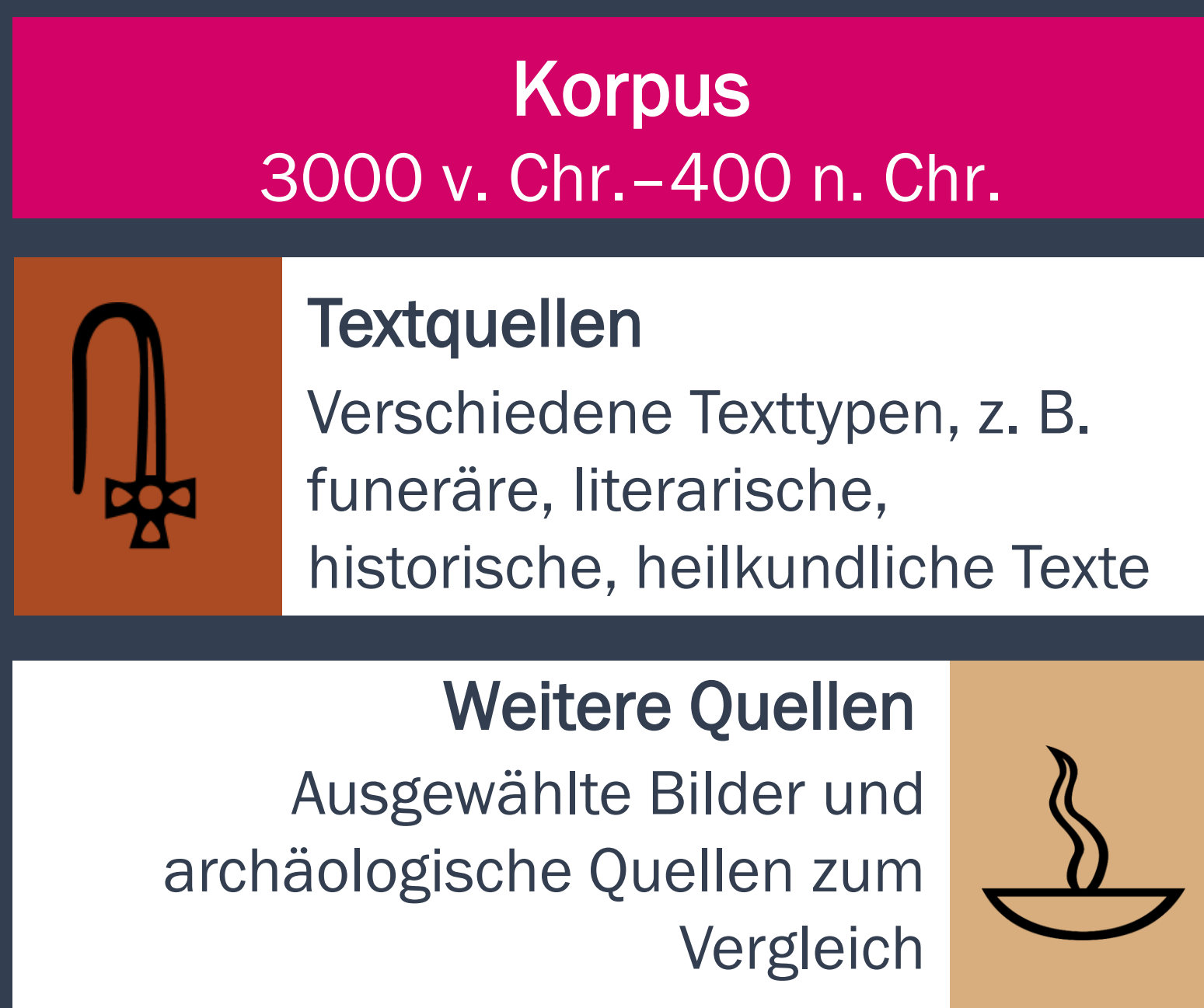
Abb. 3: Korpus.
