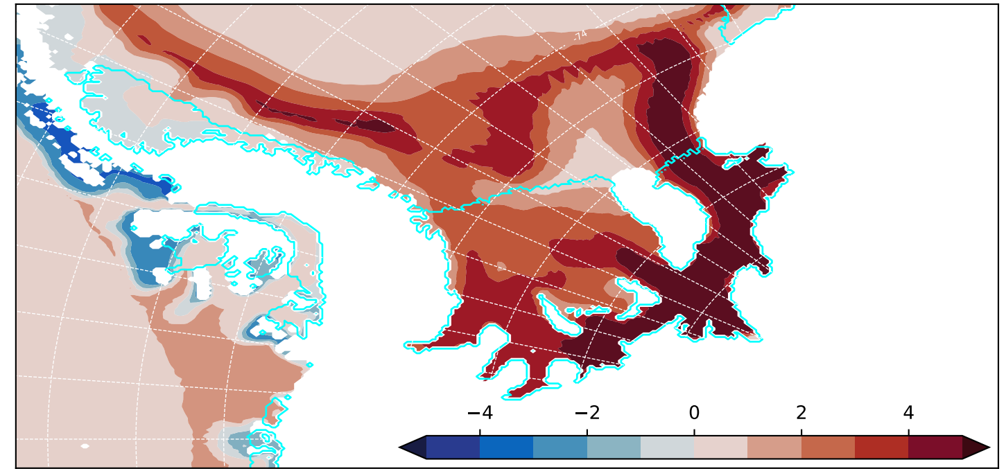
(d) Temperature anomaly, Weddell Sea (FESOM \sigma high)
