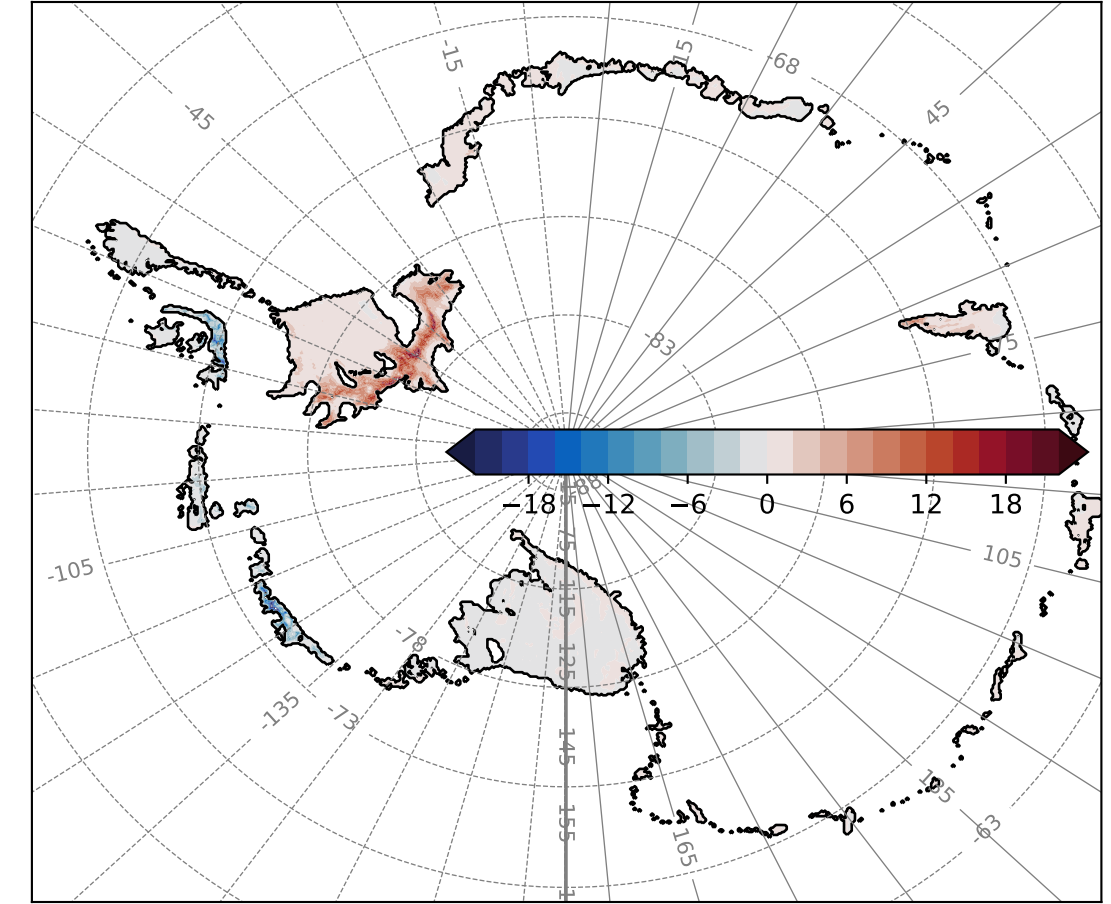
(f) Melt anomaly (FESOM z low)
