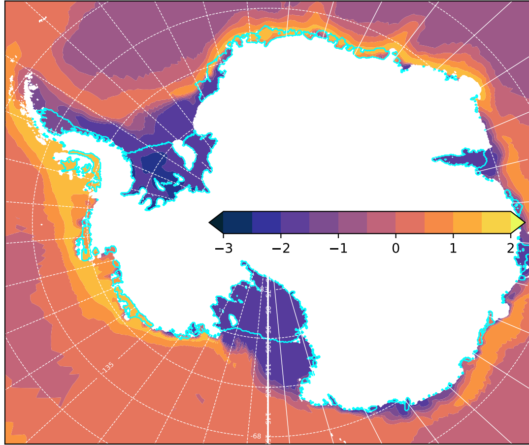
(d) Seafloor potential temperature (FESOM z low)
