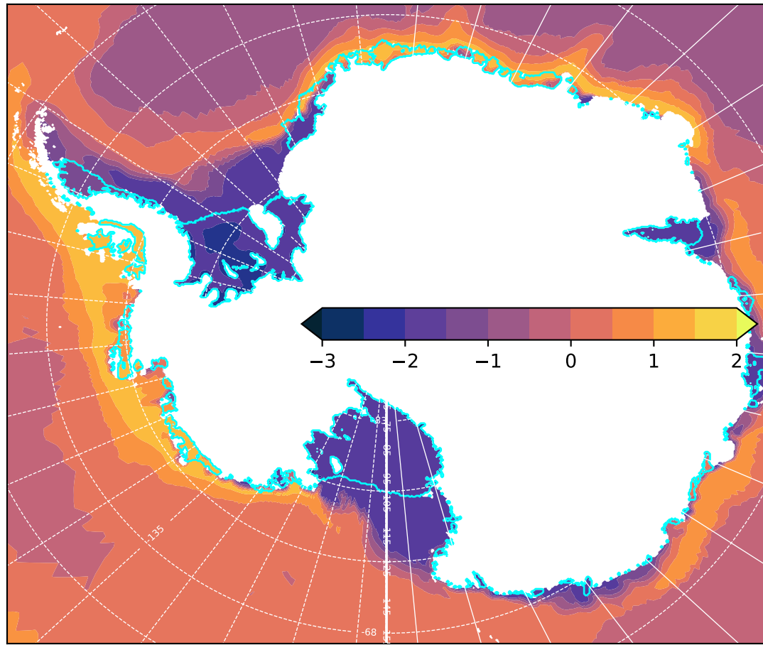
(d) Seafloor potential temperature (FESOM \sigma high)
