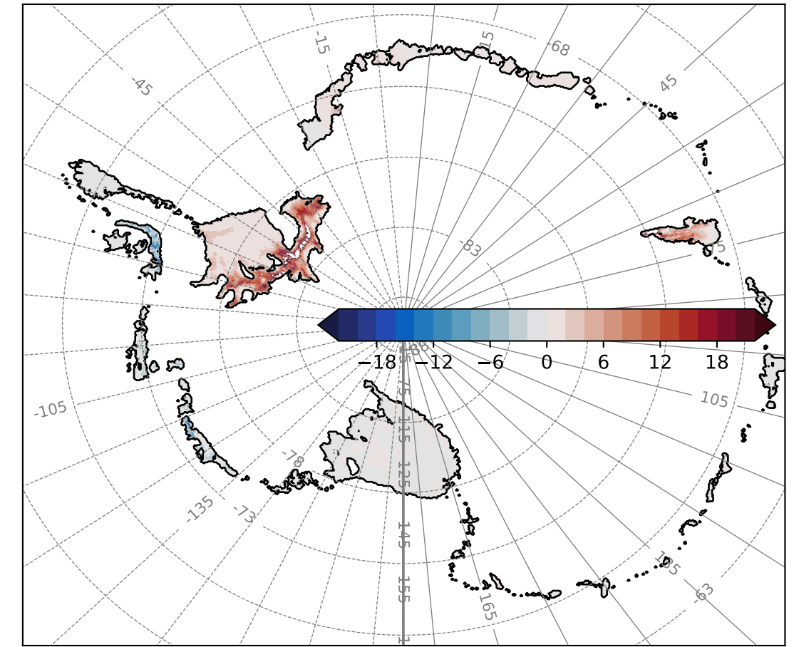
(f) Melt anomaly (FESOM \sigma high)
