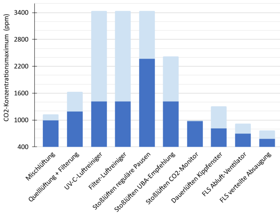
Abbildung 2: Maximale CO_2 -Konzentration in dem betrachteten Klassenraum bei Anwendung verschiedener Lüftungsmethoden unter günstigen Bedingungen (dunkelblau) oder unter ungünstigen Bedingungen (hellblau) (Tabelle 1, Anhang A.2).
