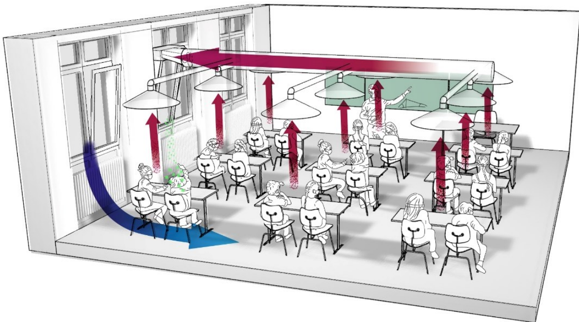
Abbildung A4: Schematische Darstellung eines Fensterlüftungssystems mit verteilter Abluftabsaugung und bodennahe Zuluft (MPIC-FLS, ventilation-mainz.de).
