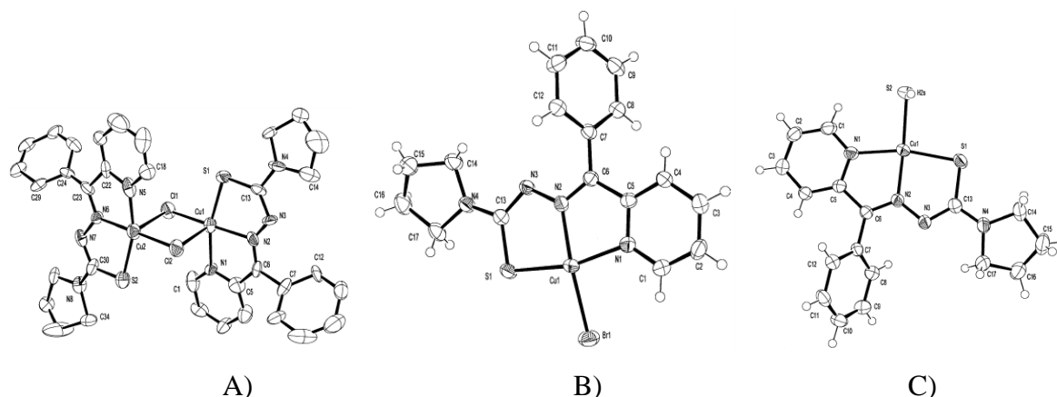
Fig.18. Structurile cristaline ale complexelor Cu(Bzpytsc4But)Cl (A), Cu(Bzpytsc4But)Br (B) și Cu(Bzpytsc4But)SH (C).
