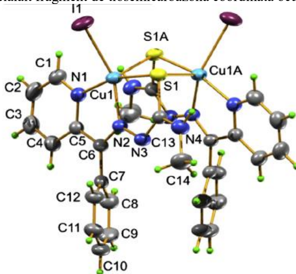
Fig.13. Structura complexului binuclear [\text{Cu}_2(\text{Bzpytsc4Me})_2\text{I}_2] .
