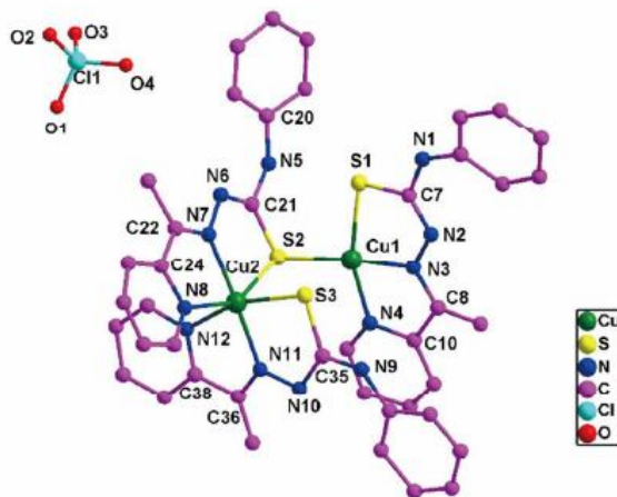
Fig.6. Structura moleculară a complexului [\text{Cu}_2(\text{Acpytsc4Ph})_3]\text{ClO}_4 .
