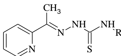
Fig.3. Schema generală a tiosemicarbazonei cu diferiți substituți în poziția N4.
