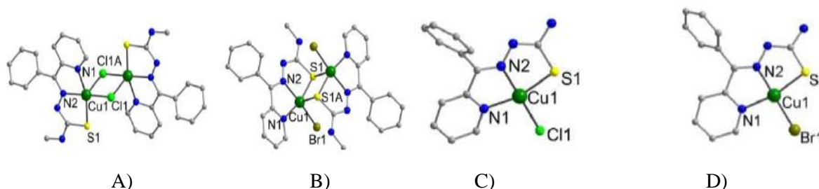
Fig.12. Structura compușilor coordinativi ai \text{Cu}(\text{II}) cu HBzpytsc și HBzpytsc4Me.
