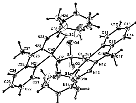
Fig.8. [\{Cu(Acpytsc4hexim)\}_2SO_4] \cdot DMF
