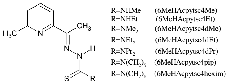
Fig.4. Schema diferitor tiosemicarbazone cu substituenți la atomul N4 ale 6-metil-2-acetilpiridinei.
