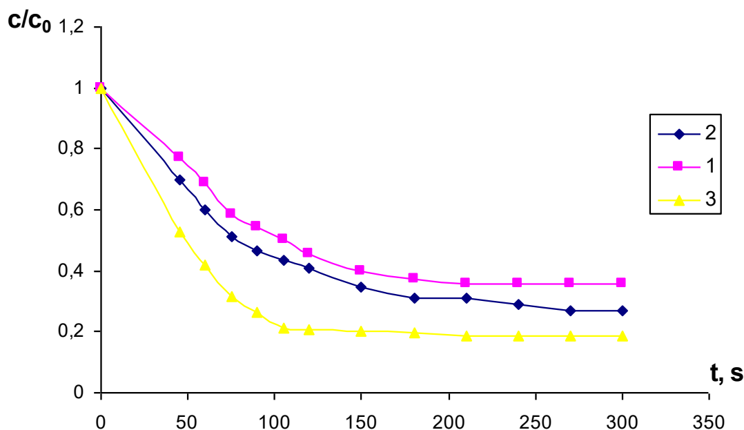
Fig.1. Gradul de decolorare a permanganatului de potasiu în sistemul KMnO_4 - FL - NaOH : 1 - [MnO_4^-] = 2,67 \cdot 10^{-4} M; 2 - [MnO_4^-] = 5,33 \cdot 10^{-4} M; 3 - [MnO_4^-] = 10,70 \cdot 10^{-4} M ( [FL] = 9,9 \cdot 10^{-4} M; [NaOH] = 0,05 M; [NaClO_4] = 0,05 M; \lambda = 525 nm; t = 25^\circ C ).
