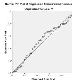
Gambar 2. Hasil Uji Normalitas Data
