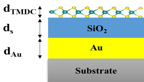
شکل ۱. ساختار مورد بررسی شامل تک لایه TMDC، لایه میانی \text{SiO}_2 ، لایه رسانای طلا و زیرلایه.
