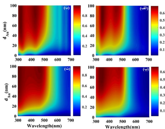
شکل ۲. جذب ساختارها بر حسب ضخامت طلا در ناحیه طول موج مرئی بدون حضور لایه میانی (الف و پ) و با حضور لایه میانی (ب و ت) (الف) Air/MoSe 2 /Au/SiO 2 (ب) Air/SiO 2 /MoS 2 /Au/SiO 2 (پ) Air/MoS 2 /Au/SiO 2 (ت) Air/SiO 2 /MoSe 2 /Au/SiO 2
