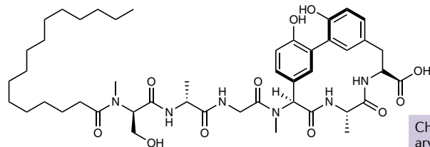
Arylomycin A-C 16
