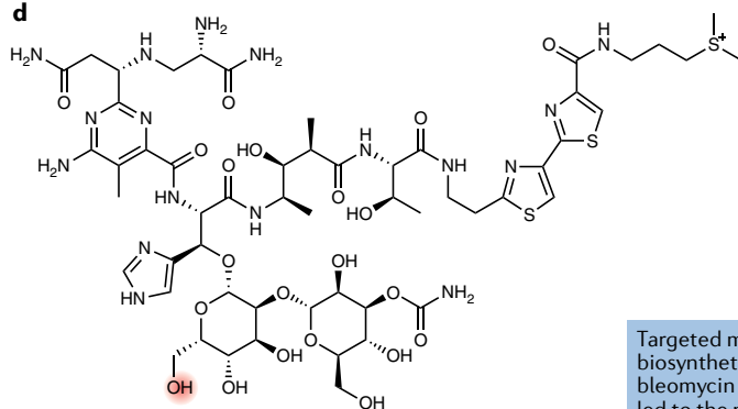
BLM A2
