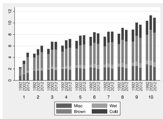
Gráfico 2: Equipamiento en los hogares según deciles de consumo eléctrico per cápita en el hogar y uso de los electrodomésticos. México 1992, 2002 y 2012.
