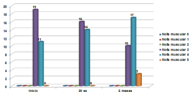
Figura 5: Fuerza musculare.
