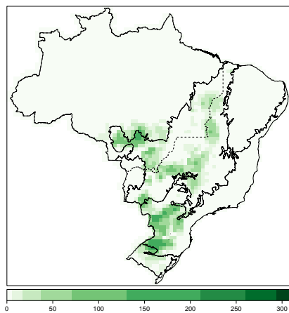
(a) Soya IBGE/PAM
