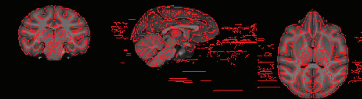
D99 edges on YRK volume
