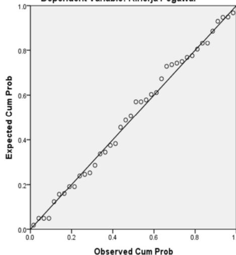
Gambar 1 Grafik Uji Normal P-P Plot
