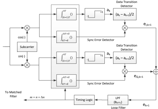
Fig. 13. Non-coherent DTTL.
