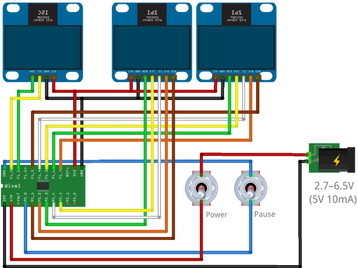
Схема підключень
