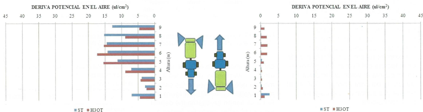
Figura 14. Perfil de deriva potencial en el aire media ( \mu\text{l}/\text{cm}^2 ) a cada lado de las calles centrales para cada tratamiento (Garcerá et al. 2018, © 2018 The Association of Applied Biologists).
