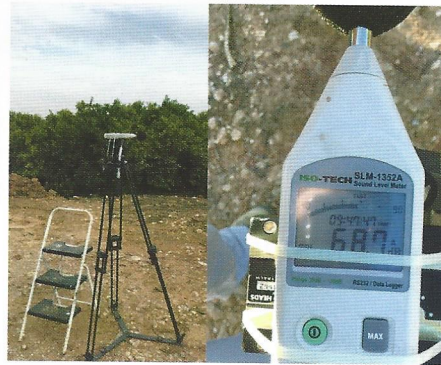
Figura 7. Sonómetro instalado para medir la contaminación acústica durante las aplicaciones.
