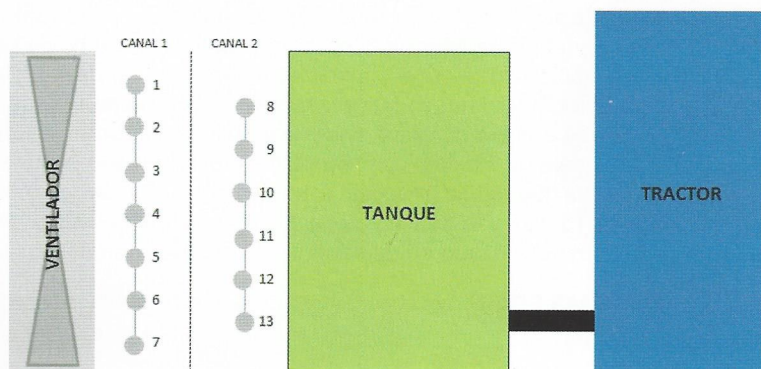
Figura 4. Localización de las boquillas en el pulverizador Fede Futur 1000L 2005.
