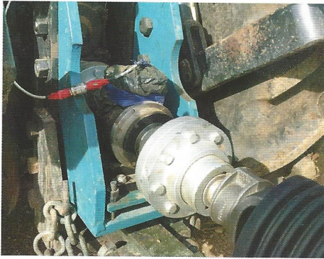
Figura 6. Sensor de par instalado en la TDF del tractor.
