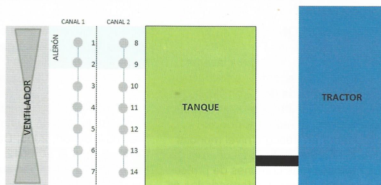
Figura 5. Localización de las boquillas en el Smartomizer Fede Futur H 3 O ® .
