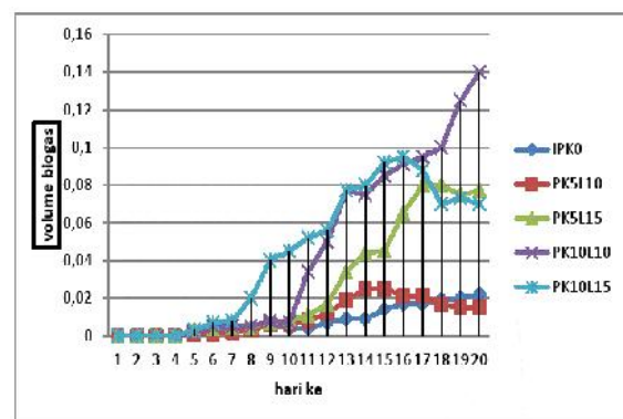
Gambar 5. Grafik Produksi Biogas
