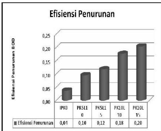
Gambar 6. Efisiensi Penurunan Kadar BOD
