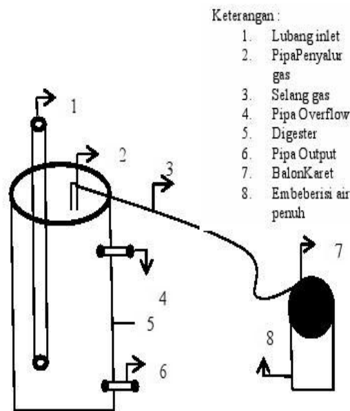
Gambar 3. Desain Alat Biogas
