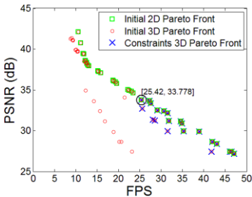
(d) 3D → 2D Pareto front of PSNR vs FPS
